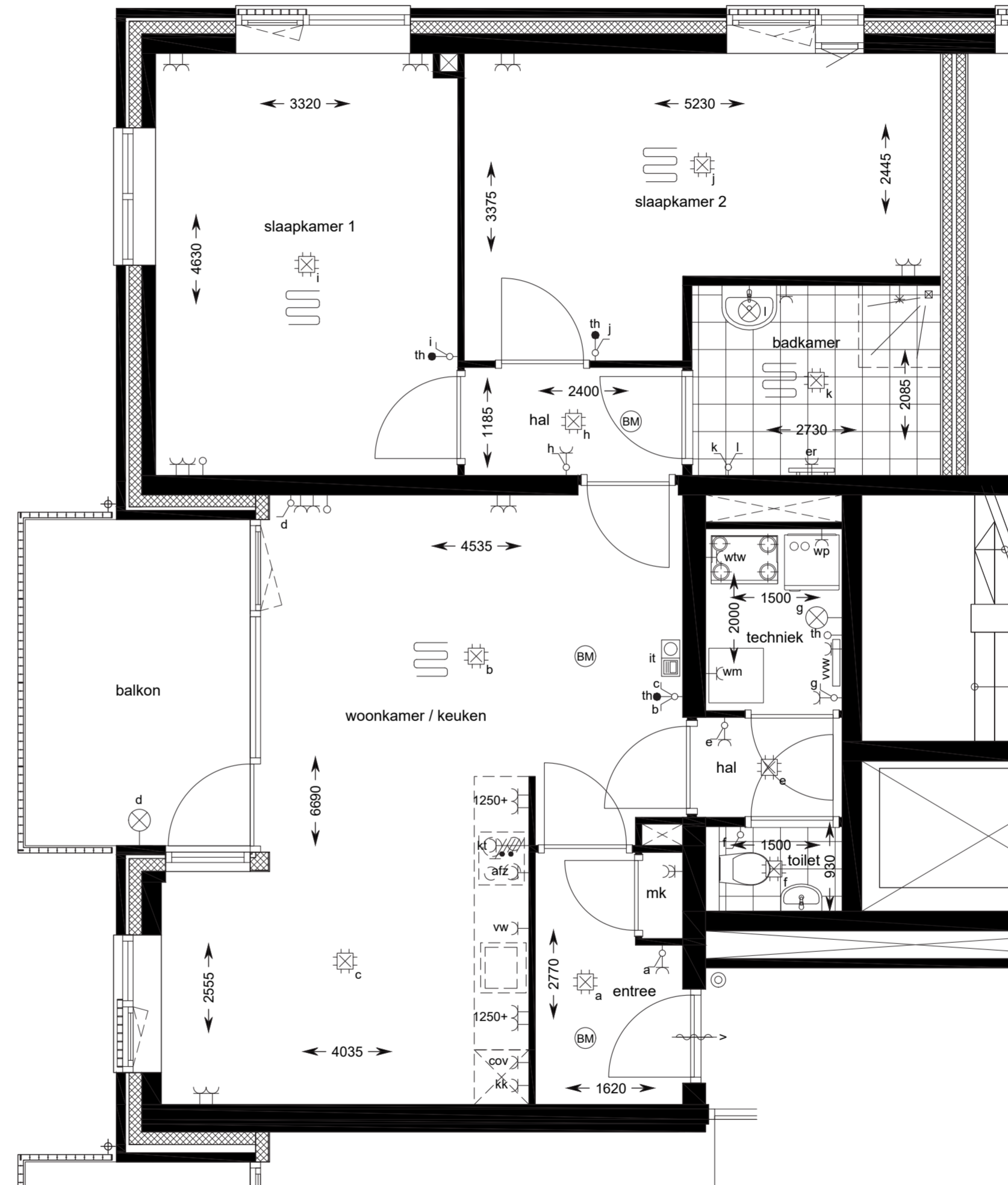
BN 46 - 2 e verdieping
