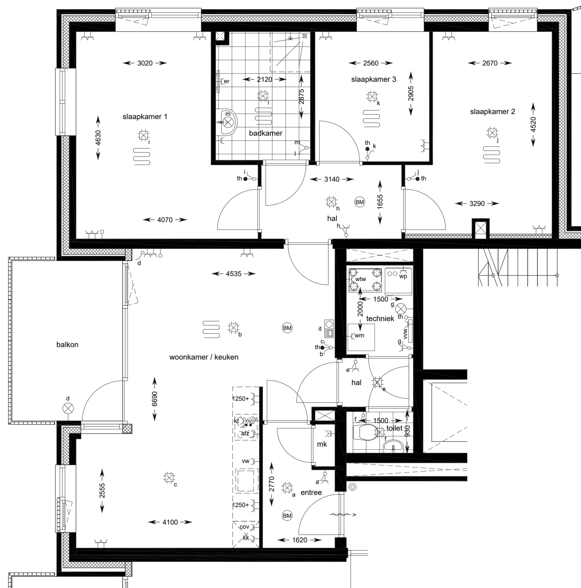
BN 50 - 3 e verdieping
